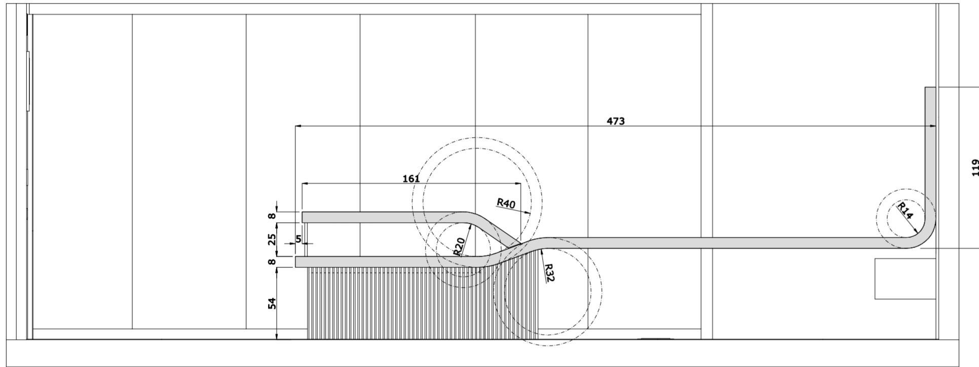
Kesit
